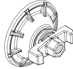
Aynalı Somun Ø120 / Anchoring Plate Nut Ø120
